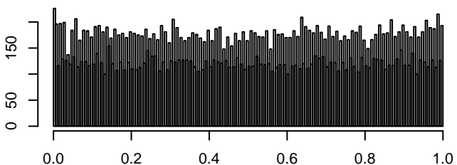
quants_lte
